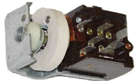
PIEZA: DS220
