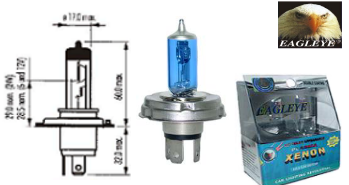
PIEZA:P45-100W-2BLUE
