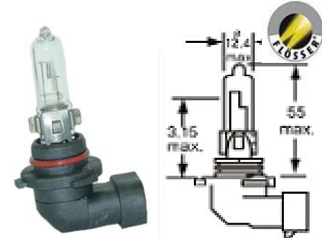
PIEZA: 9005
