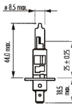
PIEZA:H1-100W-2BLUE
