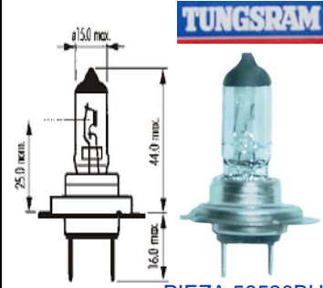
PIEZA:58520BU
