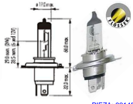
PIEZA: 92145
