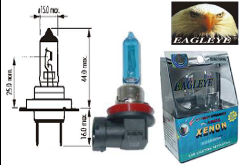
PIEZA:H7-55W-2
