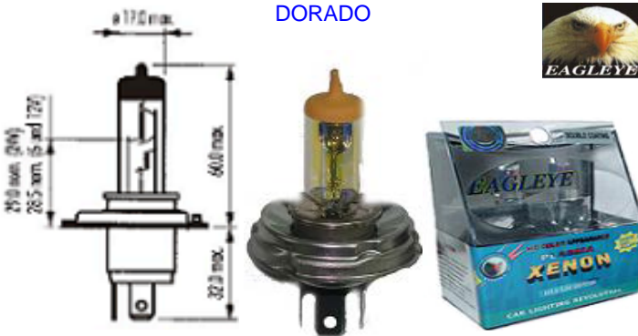
PIEZA:P43-55W-2GOLD
