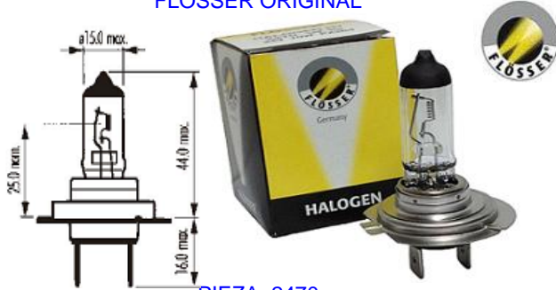
PIEZA: 2470
