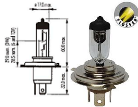
PIEZA: 925543
