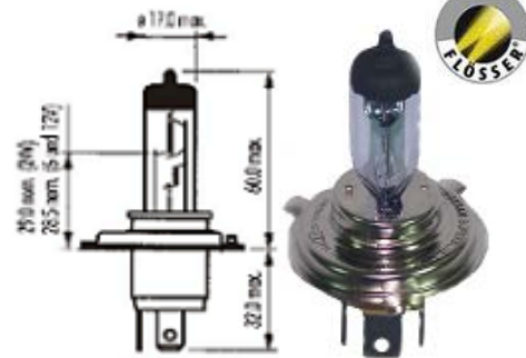
PIEZA: 8213043
