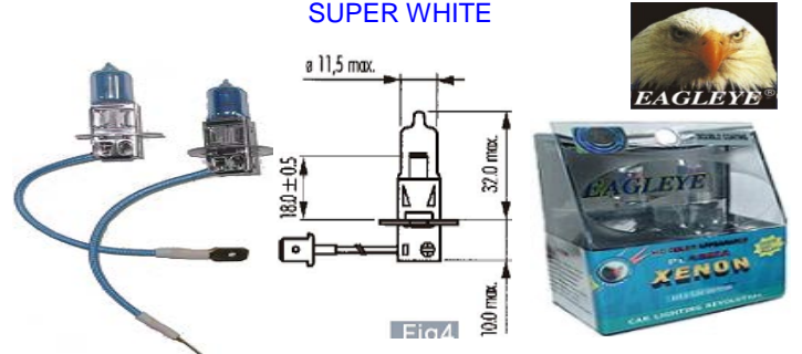
PIEZA:H3-100W-2DEEP
