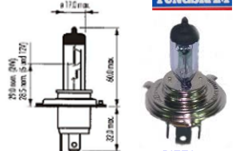
PIEZA: 52100
