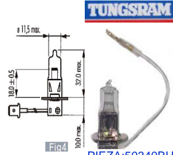
PIEZA:50340BU
