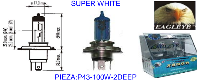
PIEZA: P43-100W-2DEEP
