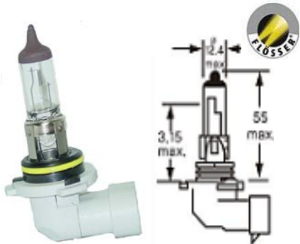
PIEZA: 9006
