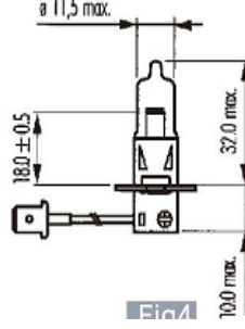
PIEZA: H3-100W-2GOLD
