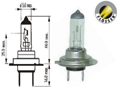
PIEZA: 2070
