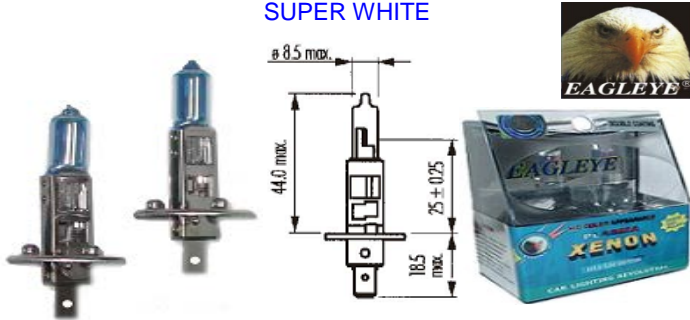
PIEZA:H1-100W-2DEEP
