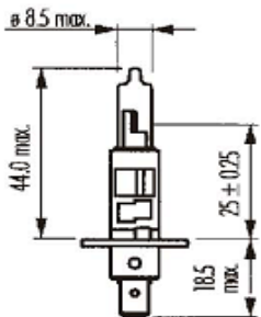
PIEZA: H1-100W-2GOLD
