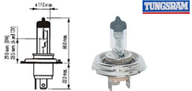
PIEZA: 52030
