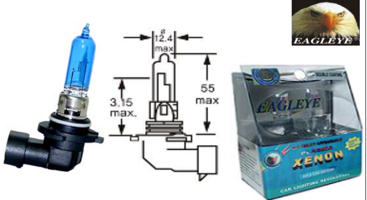
PIEZA:9005-65W-2BLUE
