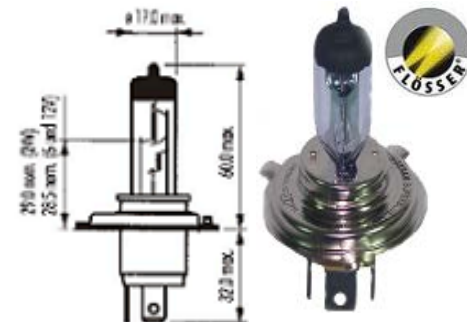
PIEZA: 8290045
