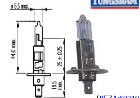
PIEZA: 50310
