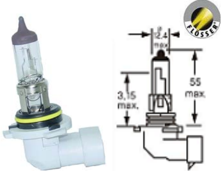
PIEZA: 9076
