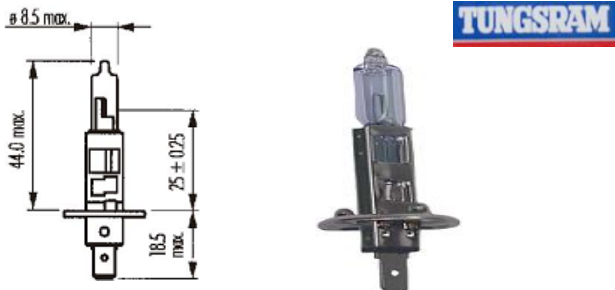
PIEZA:50320
