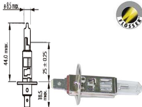
PIEZA: 3021
