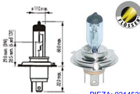
PIEZA: 9214533
