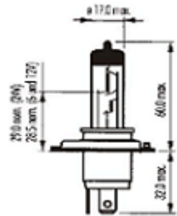
PIEZA:P43-100W-2BLUE
