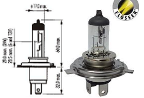
PIEZA: 725543
