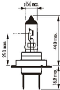
PIEZA:H7-100W-2GOLD
