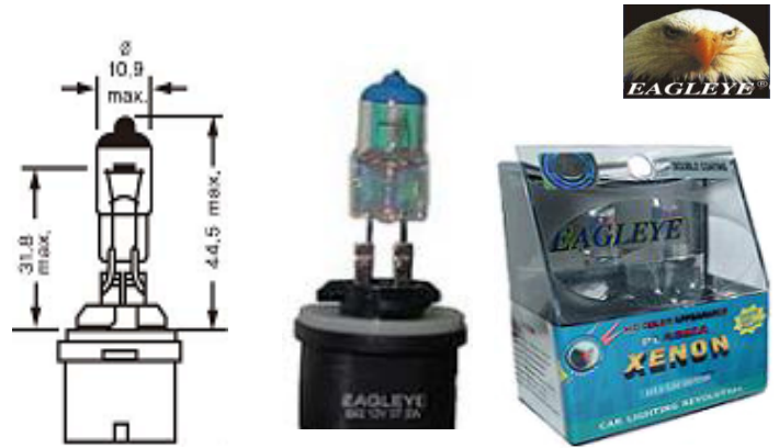
PIEZA: 893-37W-2BLUE
