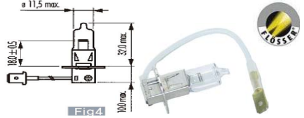
PIEZA: 13330
