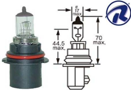
PIEZA: 9004-100W
