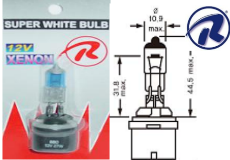
PIEZA: 880-X
