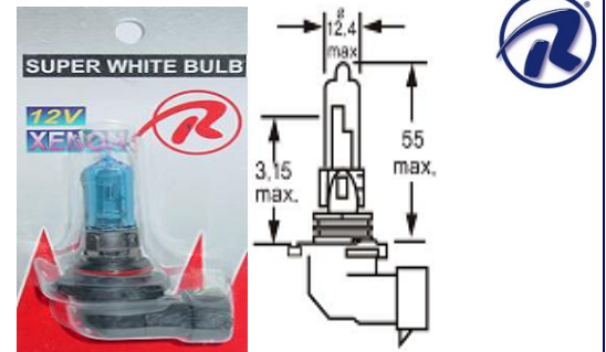
PIEZA: 9005-130W-X
