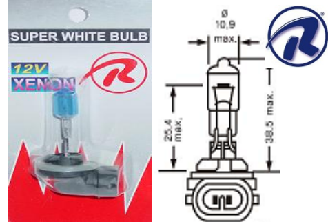
PIEZA: 889-X
