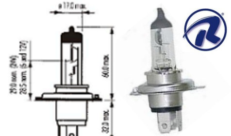
PIEZA: P43-24V-100W
