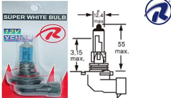
PIEZA:9006-130W-X
