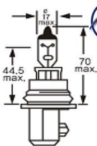
PIEZA:9004-130W
