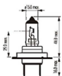
PIEZA:H7-24V-100W
