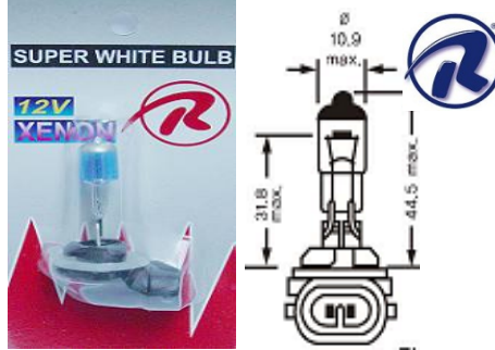
PIEZA: 881-X
