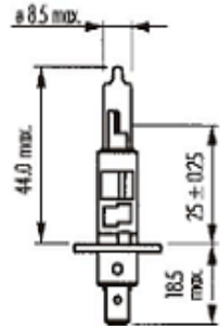
PIEZA:H1-24V-100W
