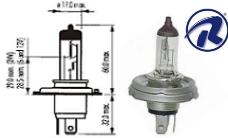
PIEZA: P45-24V-100W
