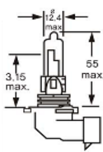
PIEZA:9005-130W
