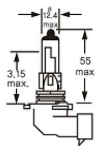
PIEZA:9006-130W
