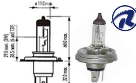
PIEZA: P45-24V-75W
