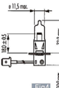
PIEZA:H3-24V-100W
