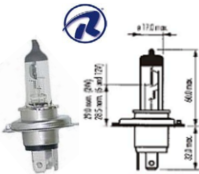
PIEZA: H4P43T
