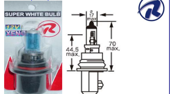
PIEZA: 9007-130W-X
